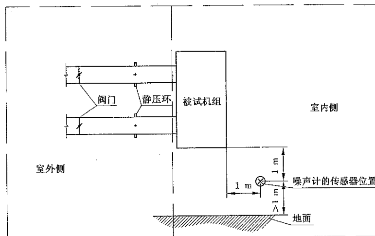
图 G.1 壁挂式机组
