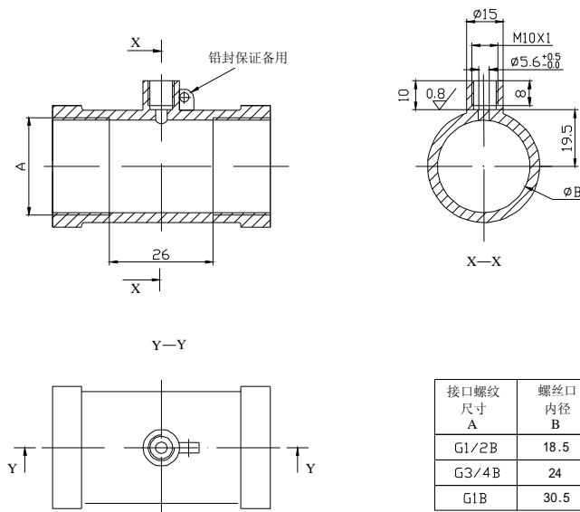
图 C11 探头的焊接接头和密封垫
