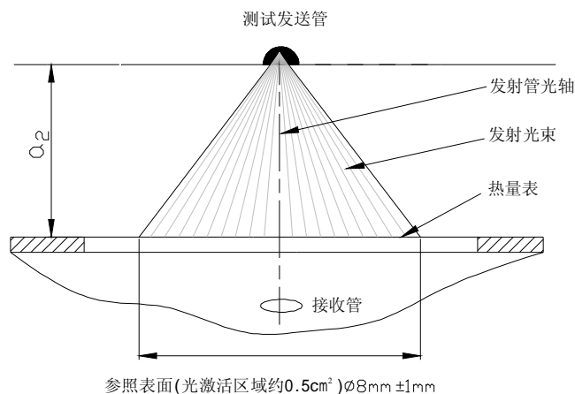
图 B7 接收管的测试示意图
