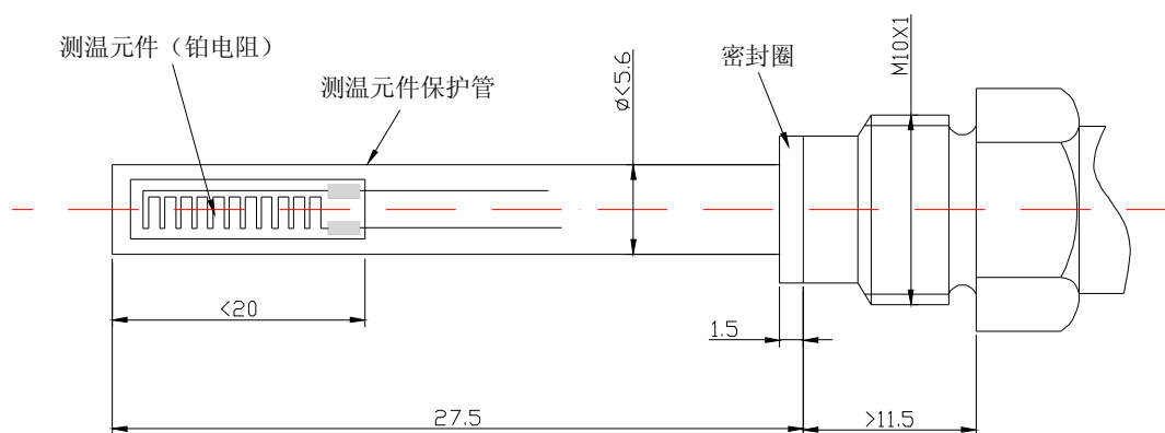
图 C1 DS 型测温探头结构
