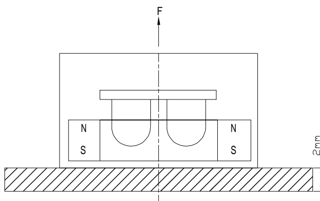
图 B3 吸引力示意图
