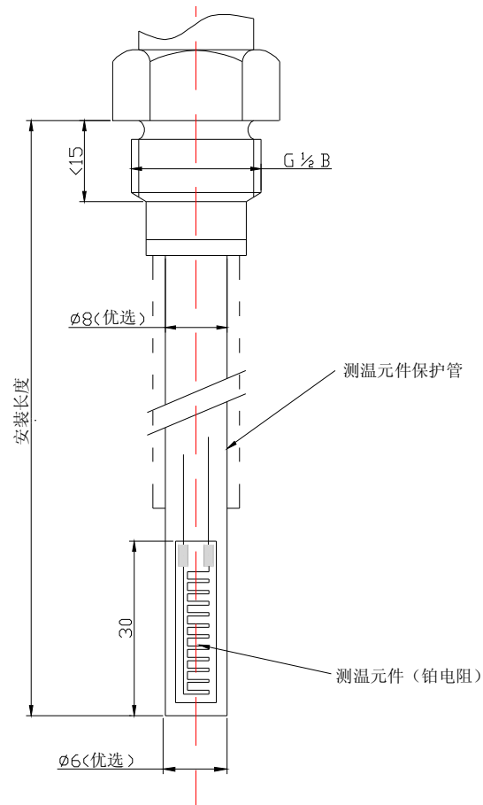
图 C6 DL—电缆型，直接插入、长型探头
