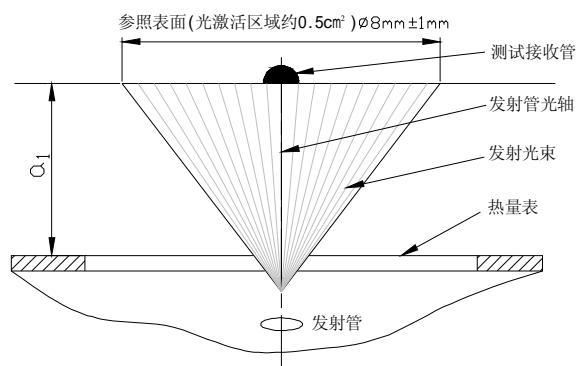
图 B6 发射管的测试示意图
