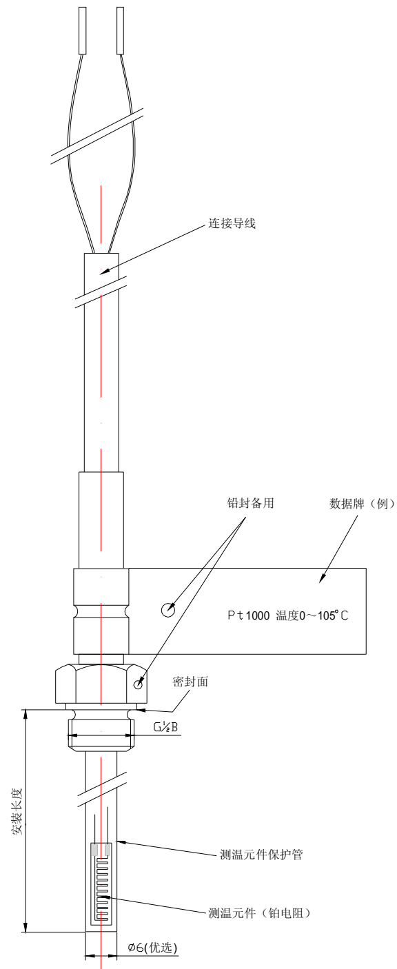
图 C8 DL- 电缆型,直接插入,长型探头
