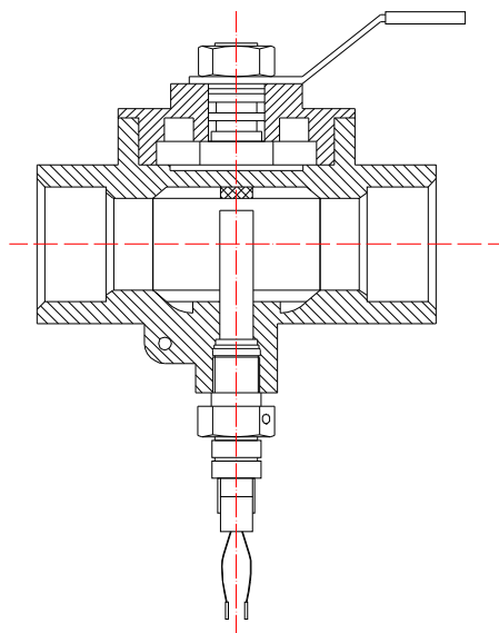
图 C7 直接插入球阀DS型探头
