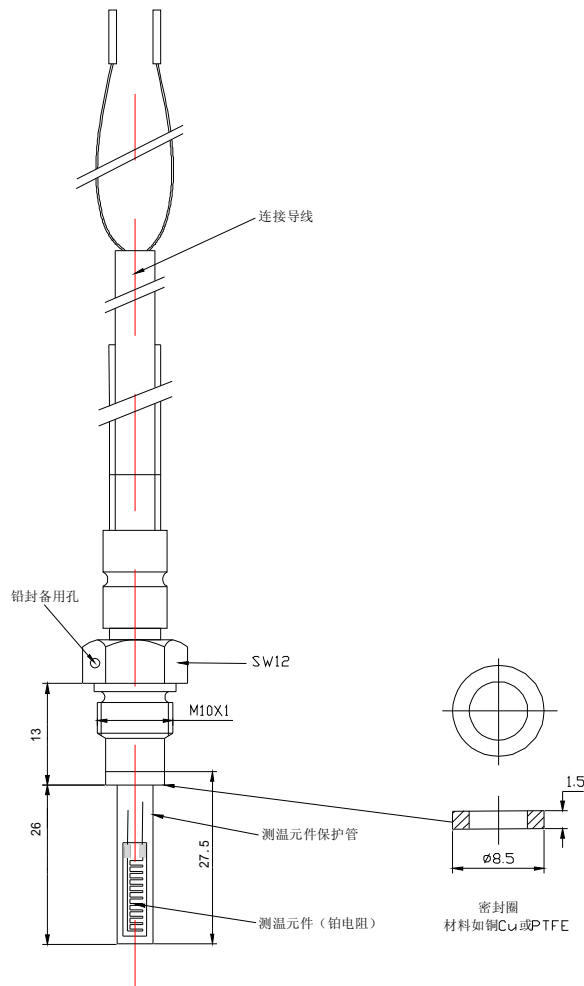
图 C5 DS-电缆型,直接插入,短型探头
