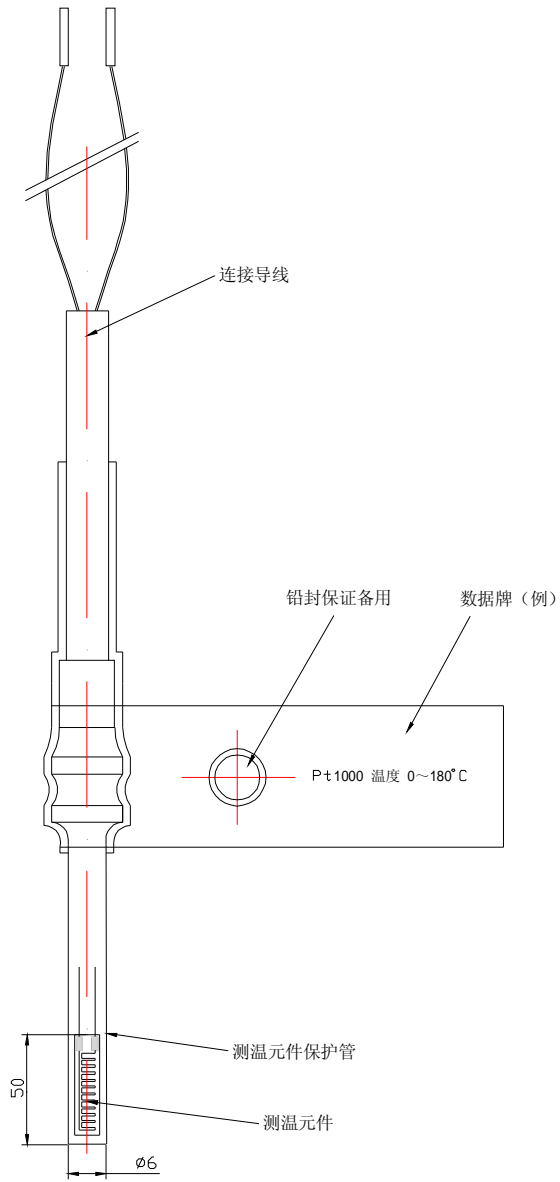
图 C10 PL - 电缆型, 插入套管式探头
