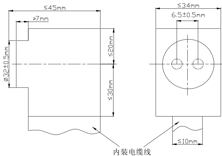
图 B2 读写头的尺寸图
