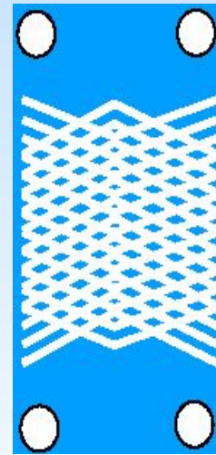
H + H = L 型通道水流示意 特点：K较大，阻力较大
