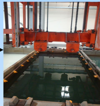
水洗处理
