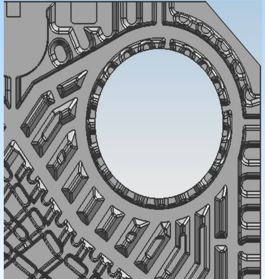
其它公司板片出水口
